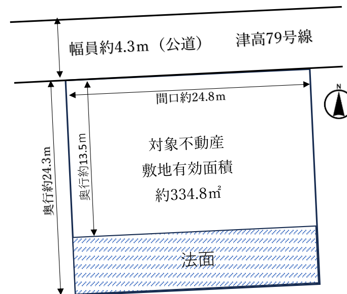
【区画図】
